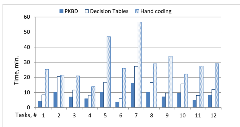
Рисунок 14 – Результаты сравнения PKBD, таблицы решений и ручное кодирование по временному критерию
