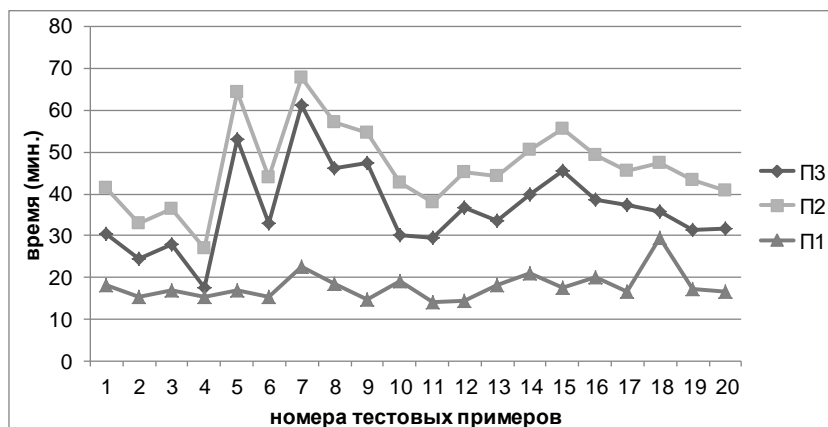
Рисунок 12 – Результаты оценки временных затрат на разработку БЗ разными подходами: П1 – концептуальное моделирование + KBDS/PKBD; П2 – концептуальное моделирование + CLIPSWin; П3 – CLIPSWin
