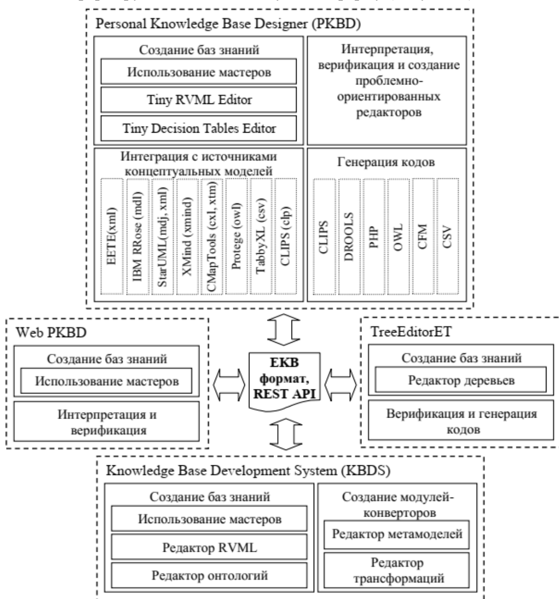
Рисунок 6 – Структура комплекса программных систем с указанием основных функций и подсистем
